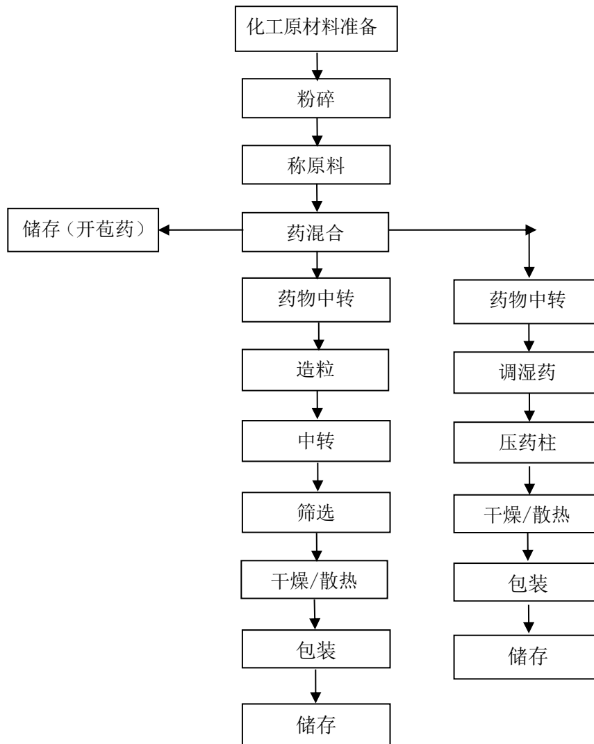
图 2.3-2 药物裸药效果件（亮珠、药柱、开苞药）生产工艺流程图
