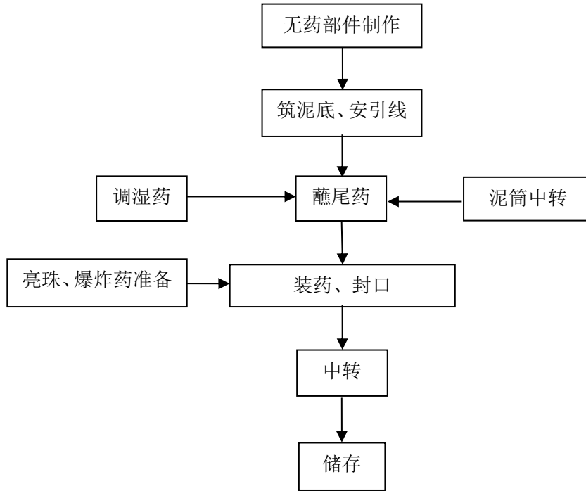
图 2.3-1 效果件内筒生产工艺流程图
