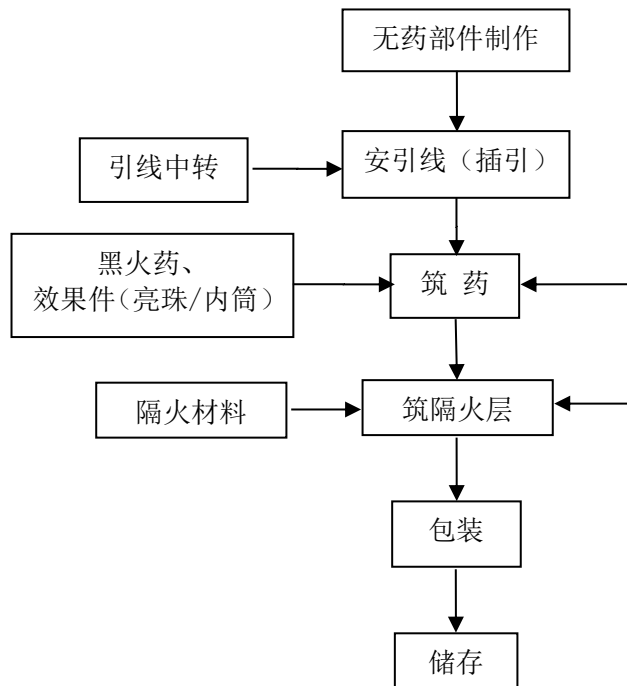
图 2.3-4 吐珠类产品生产工艺流程图
